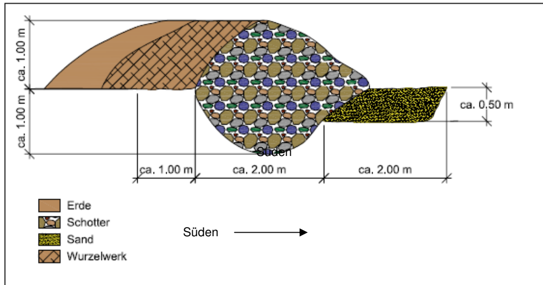
Abb. 19: Querschnitt durch einen Steinriegel für Echsenbiotope. (Zeichnung: RIK- Daniela Gaede)
