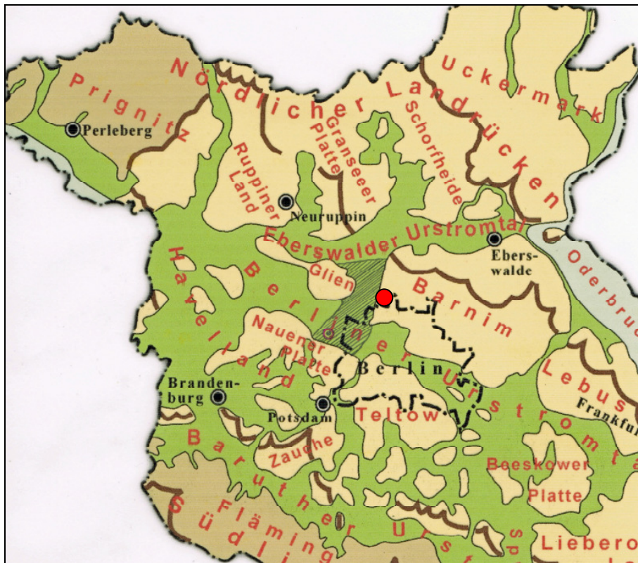
Abb. 12: Geomorphologische Lage von Schönfließ (rote Markierung) im Grenzbereich der Spandau-Oranienburger Havelniederung (graue Schraffur) und dem Westbarnim. (Quelle RIK: gestaltet nach : SCHULTZE 49 ).
