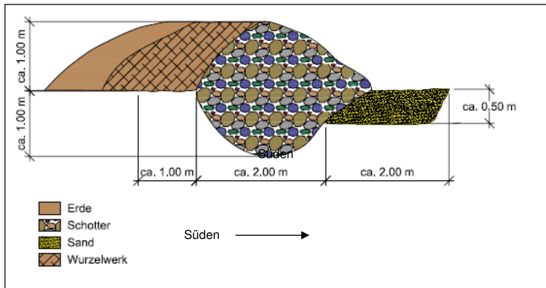
Abb. 17: Querschnitt durch einen Steinriegel für Echsensbiotope. (Zeichnung: RIK- Daniela Gaede)
