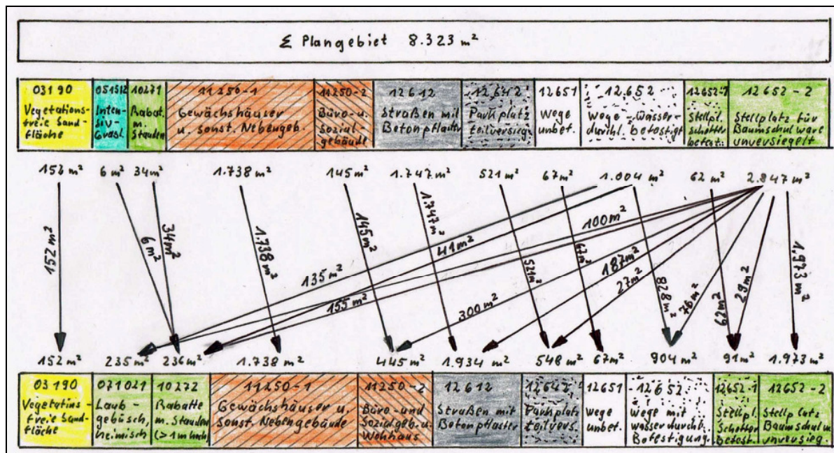
Abb. 16: Netzwerkmodell der Eingriffs- und Ausgleichsmaßnahmen bezüglich der Flächenwanderungen von den Ausgangsbiotopen vor dem Eingriff zu den Zielbiotopen nach dem Eingriff.
